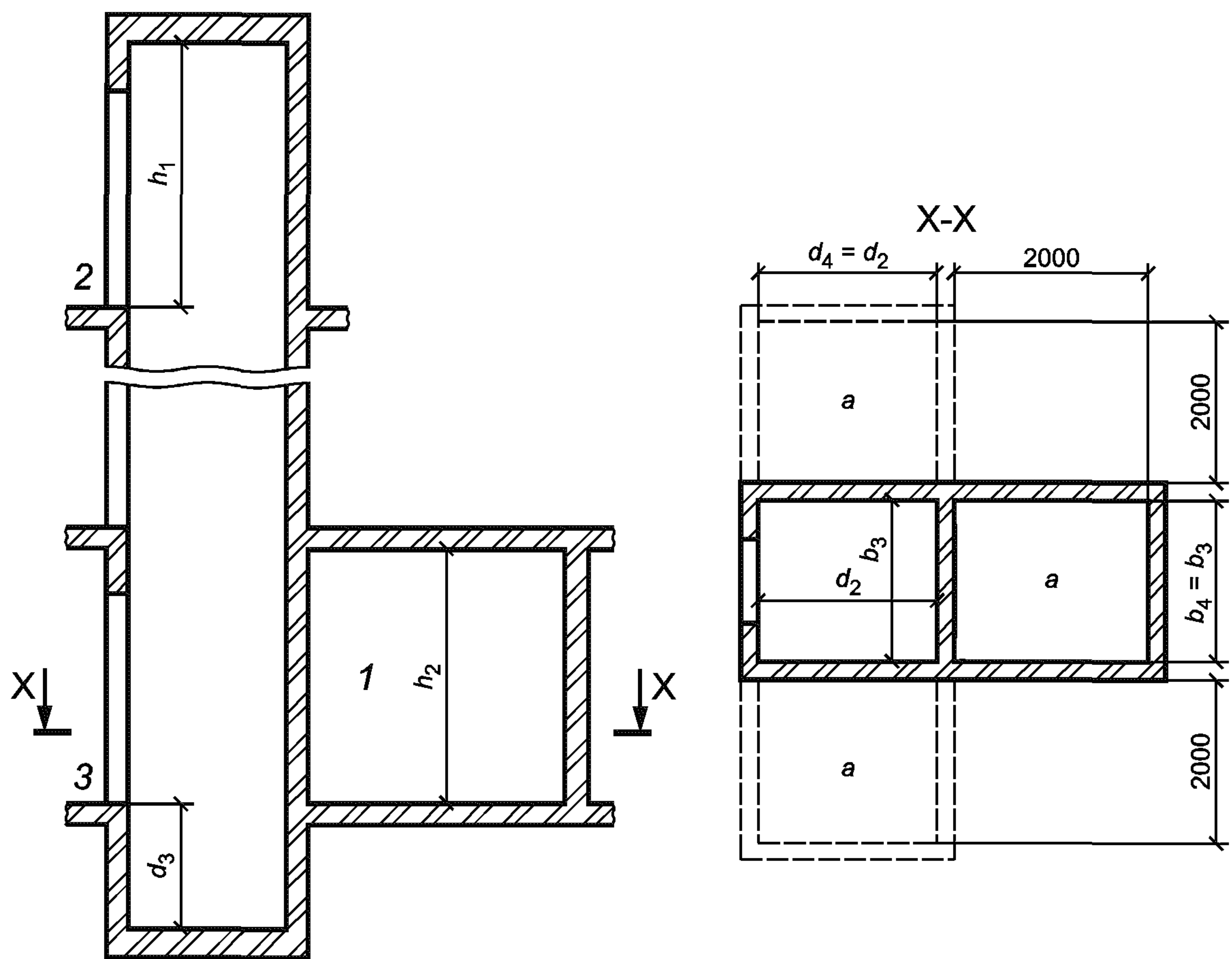
a — машинное помещение (вход в машинное помещение не показан); b_3 — ширина шахты; b_2 — ширина машинного помещения; d_2 — глубина шахты; d_3 — глубина прямка; d_4 — глубина машинного помещения; h_1 — расстояние от уровня верхней остановки до перекрытия шахты; h_2 — высота машинного помещения; 1 — машинное помещение; 2 — верхняя остановка; 3 — нижняя остановка
