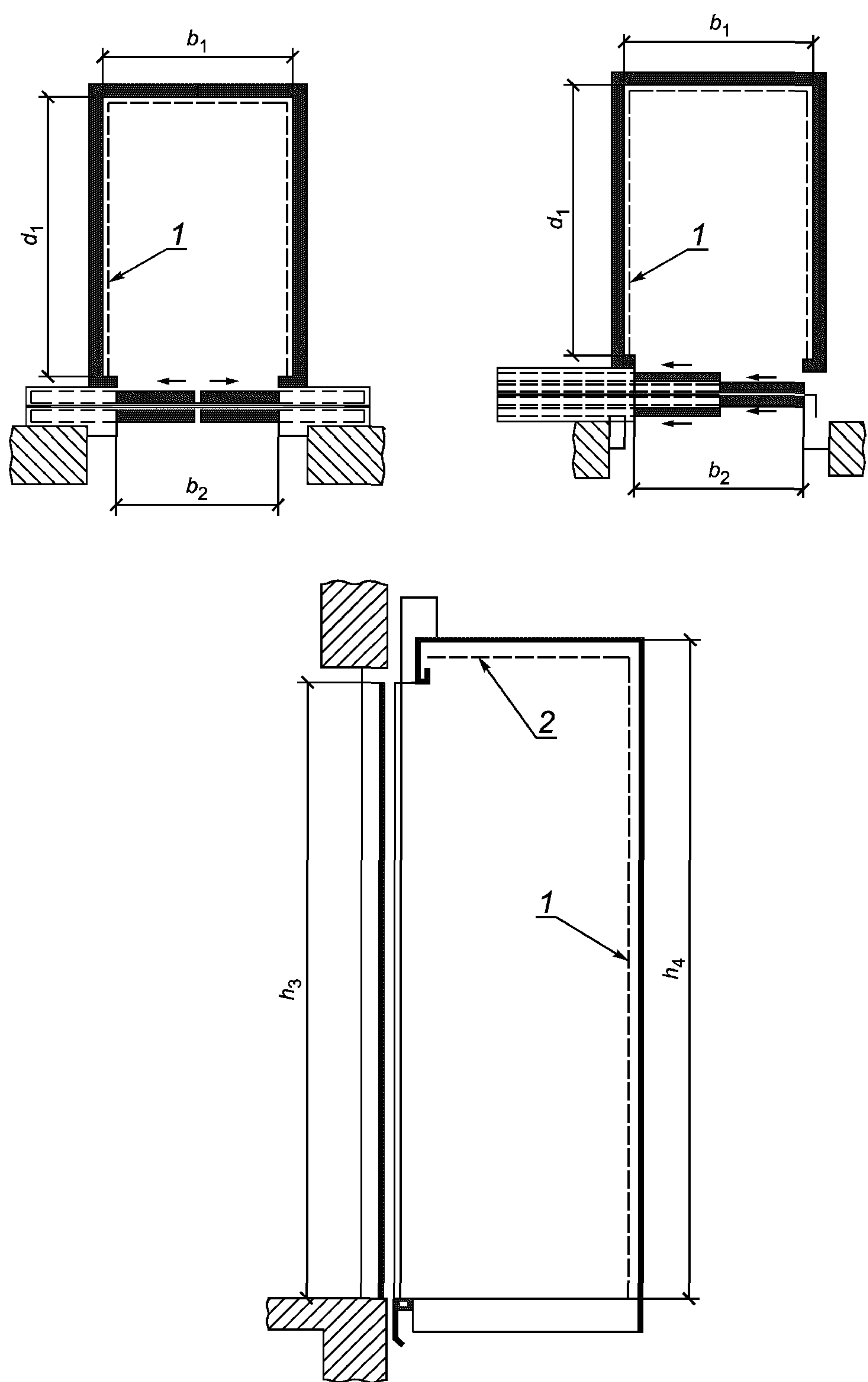
b_1 — ширина кабины; b_2 — ширина дверного проема; d_1 — глубина кабины; h_3 — высота дверного проема; h_4 — высота кабины 1 — облицовка купе кабины; 2 — подвесной потолок
